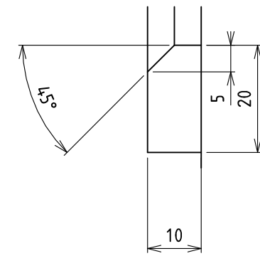
Profil lišty
